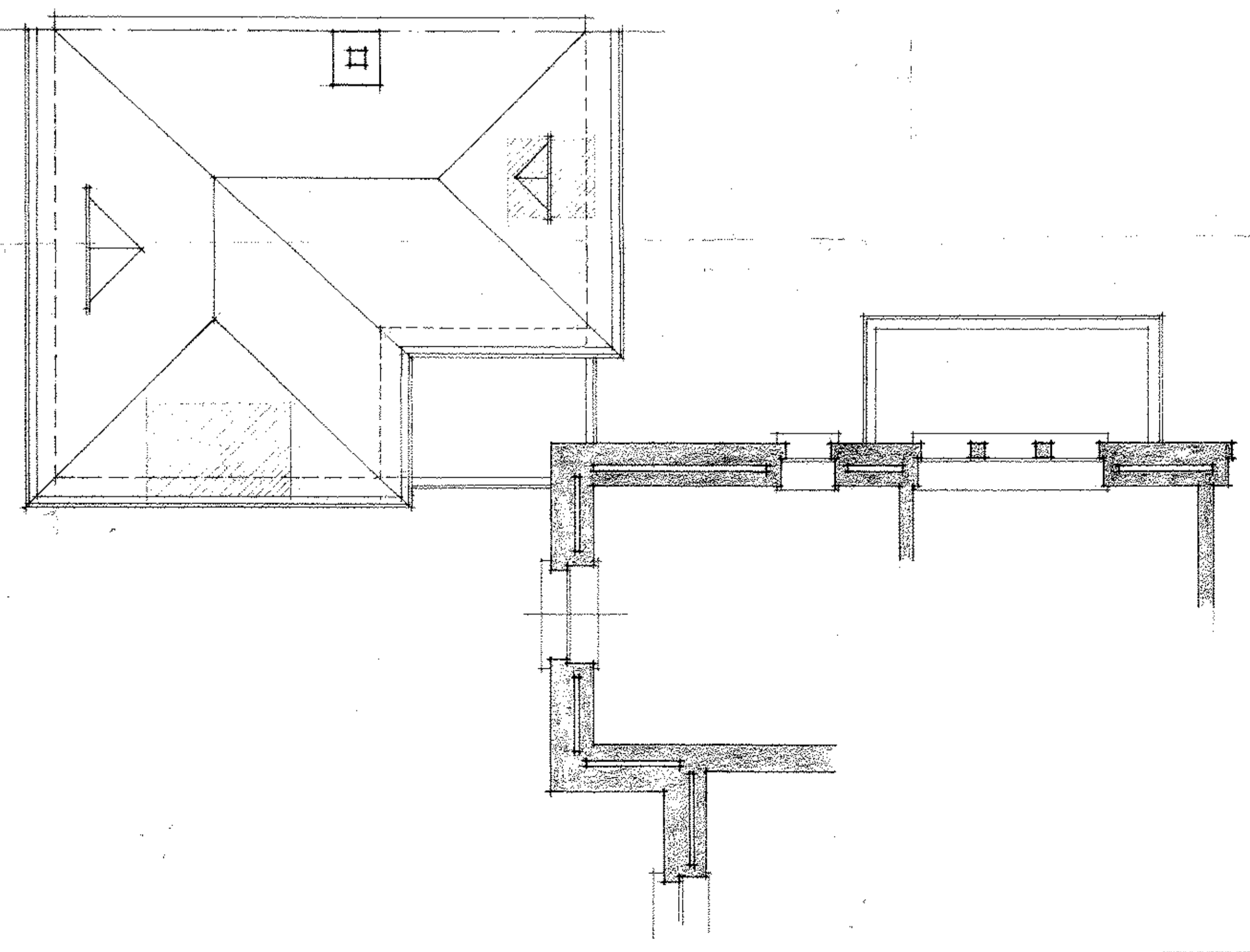
PLAN DU 1ER ETAGE
